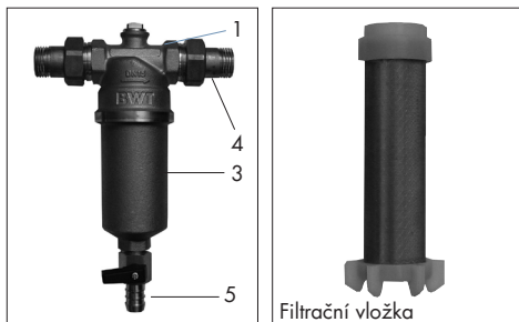
Filtrační vložka
