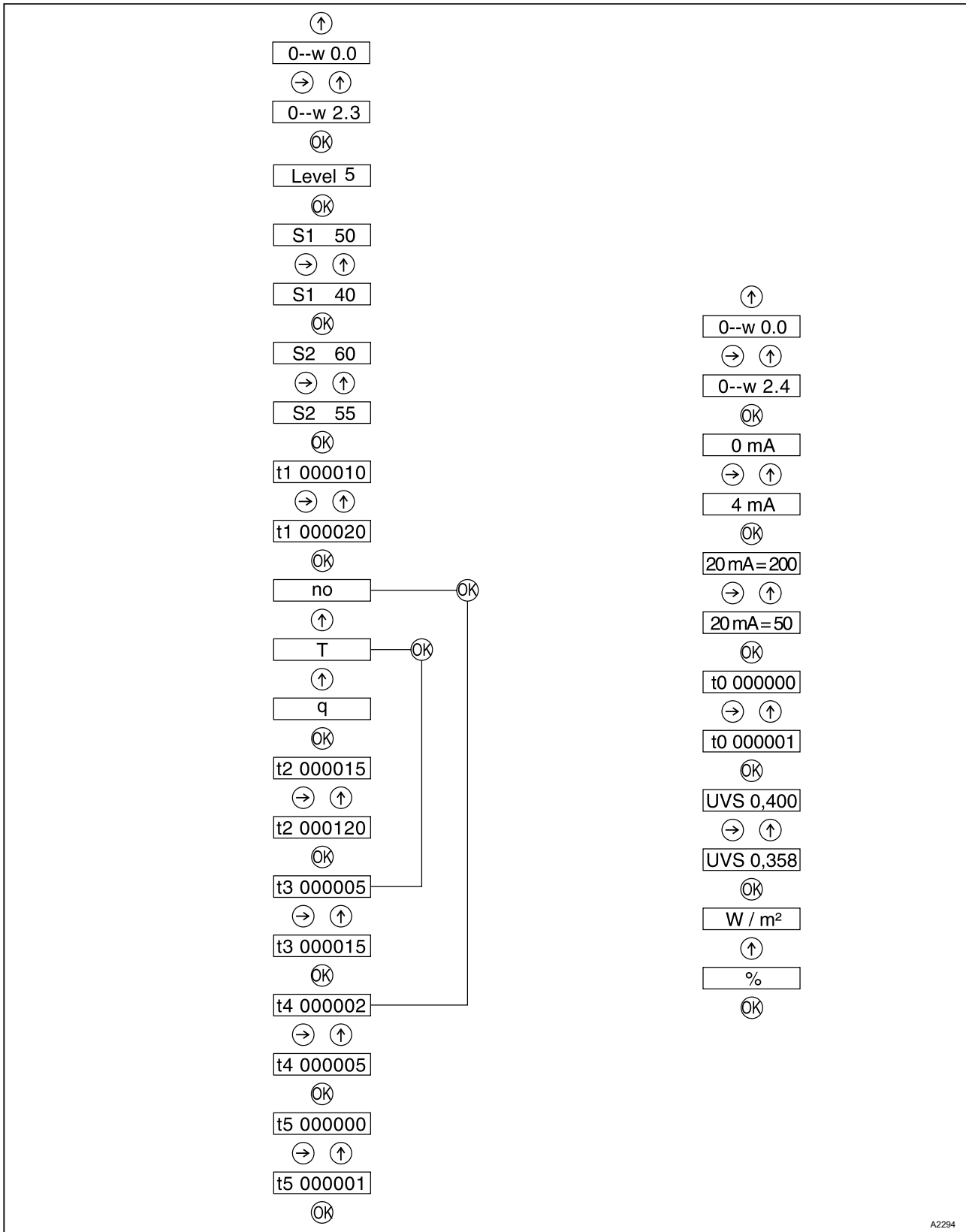
Abb. 3: Programmierschema
