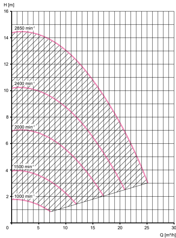
Hydraulische curven BWT EUROSTAR III Eco Touch Pro
