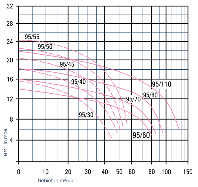
Hydraulische curven Badu 95
