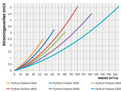
Drukverliezen van de Python Polaire filters met filtratiebelasting
